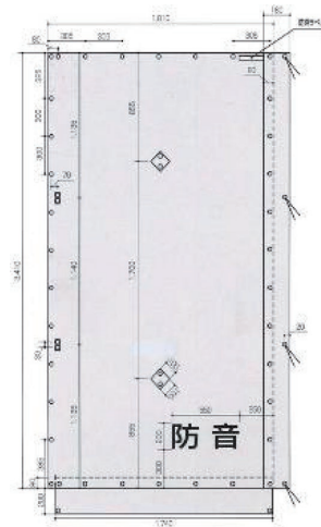
製品仕様図(0.67mm品)
